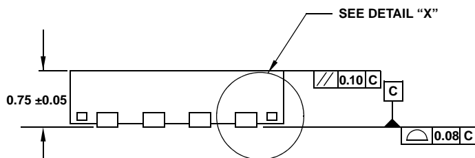
側面図
